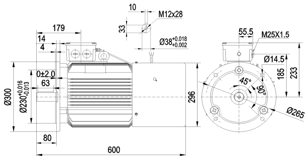
YEB4-132S 5.5kW(96kg)
