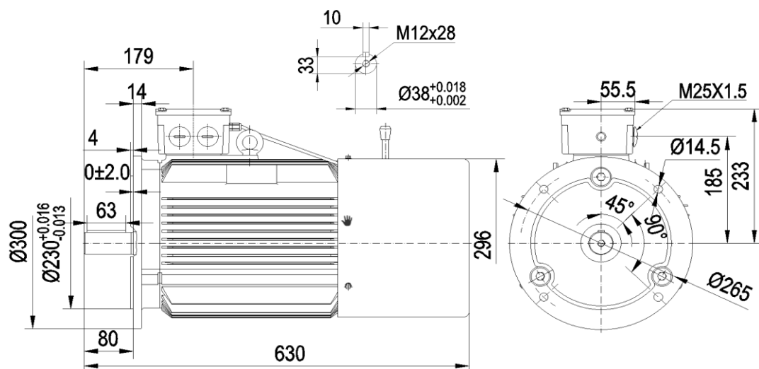
YEB4-132M 7.5kW(105kg)
