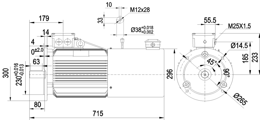
YEB4-132M 7.5kW(105kg)
