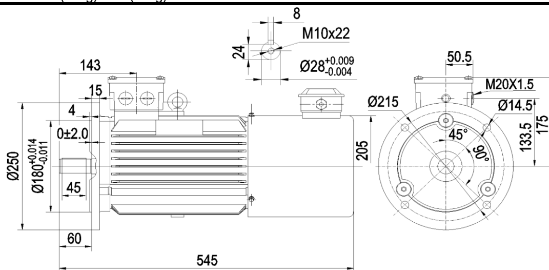
YE4-100L 2.2kW(56kg)/3kW(60kg)
