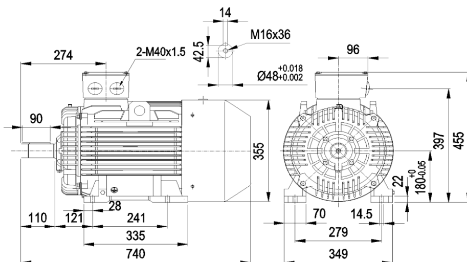
YE4-180M 18.5kW(205kg)
