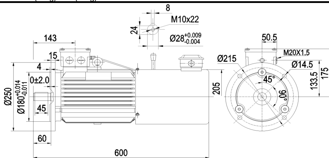
YEB4-100L 2.2kW(61kg)/3kW(65kg)
