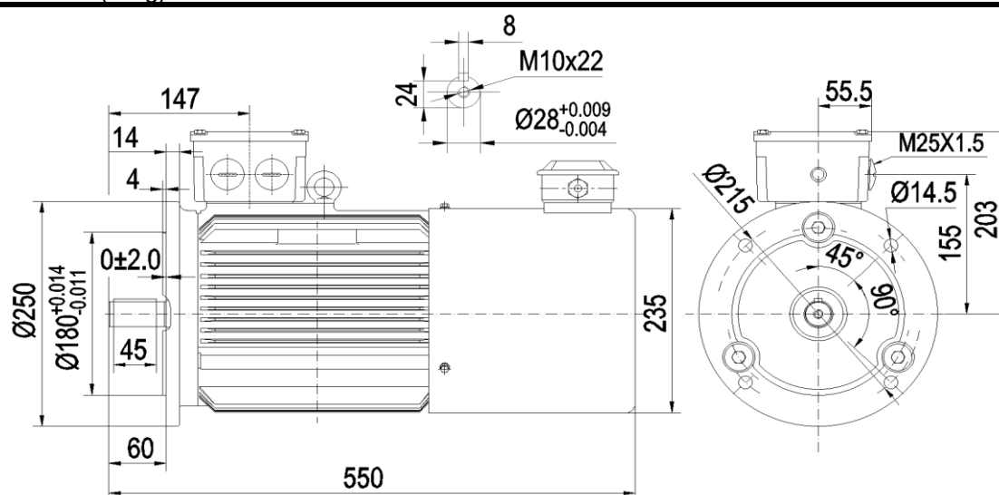
YE4-112M 3.7kW(67kg)
