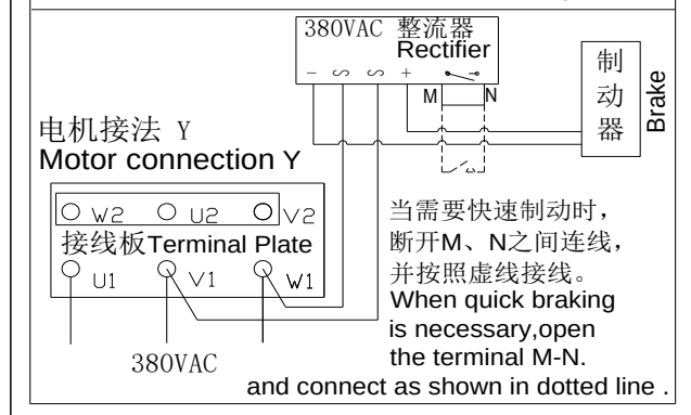
接 线 图 Connection Diagram
