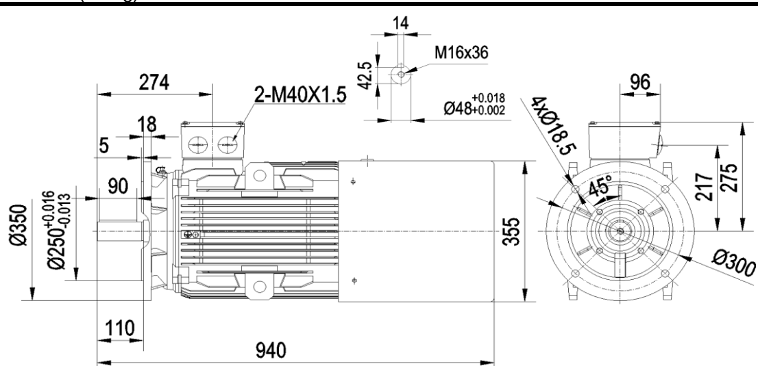
YEB4-180L 22kW(268kg)
