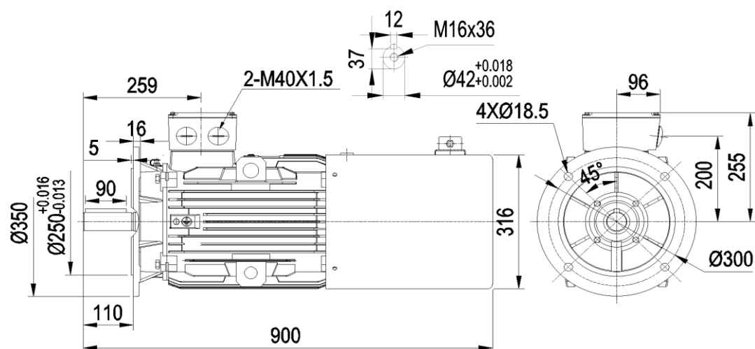
YEB4-160L 15kW(186kg)
