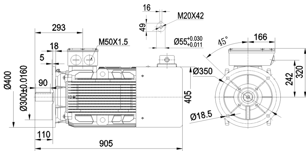
YE4-200L 30kW(270kg)
