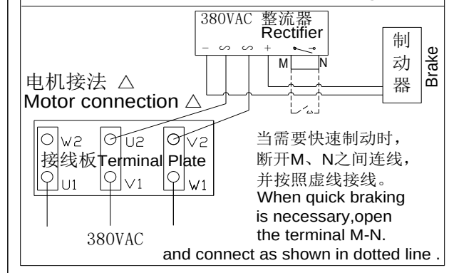
接 线 图 Connection Diagram
