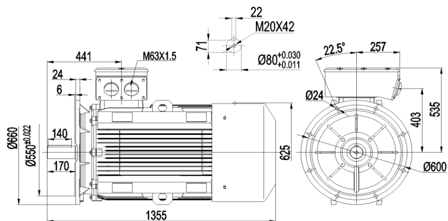
YE4-315M/YE4-315L1 132kW(1070kg)/160kW(1185kg)
