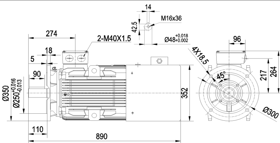
YE4-180L 22kW(240kg)
