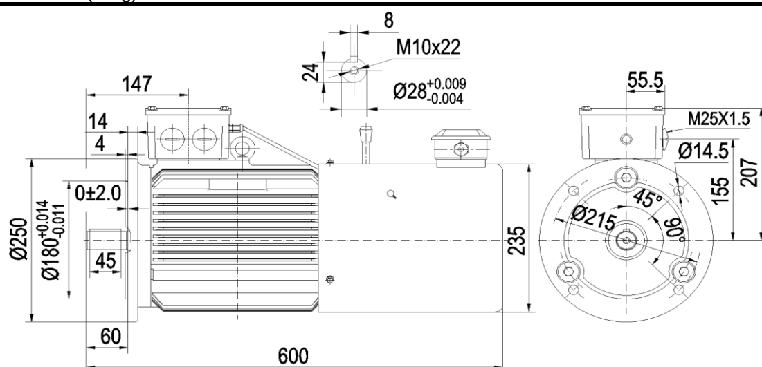
YEB4-112M 3.7kW(74kg)
