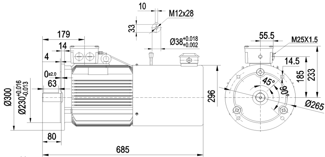
YEB4-132S 5.5kW(96kg)
