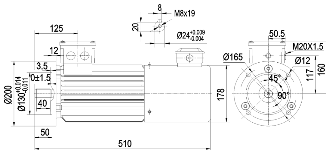
YE4-90L 1.5kW(45kg)
