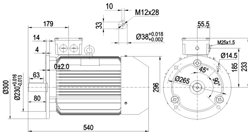
YE4-132M 7.5kW(95kg)
