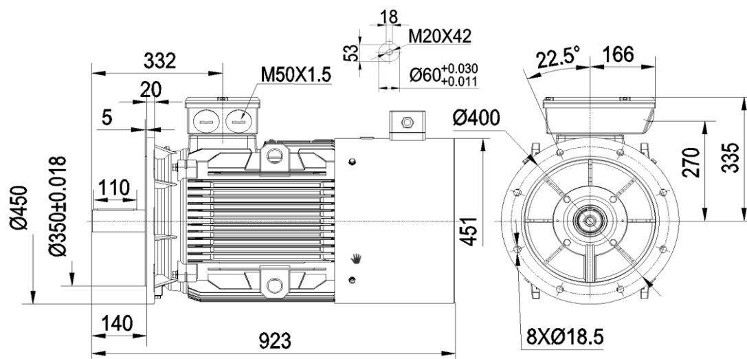
YE4-225S 37kW(360kg)
