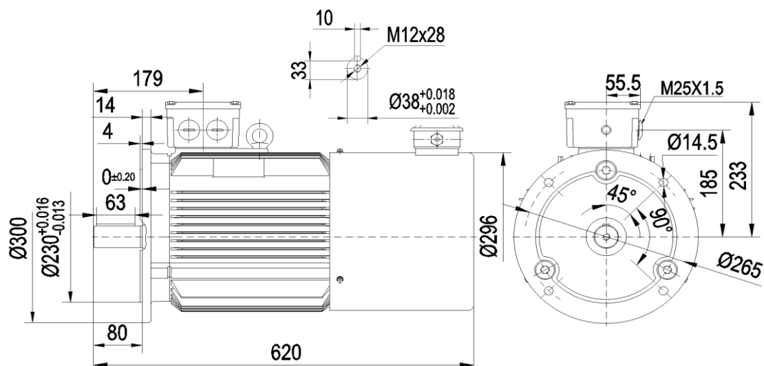
YE4-132S 5.5kW(86kg)
