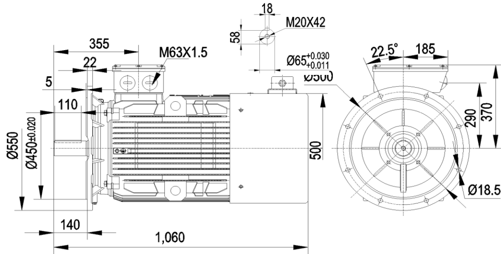
YE4-250M 55kW(480kg)
