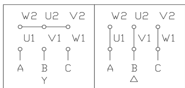
接 线 图
