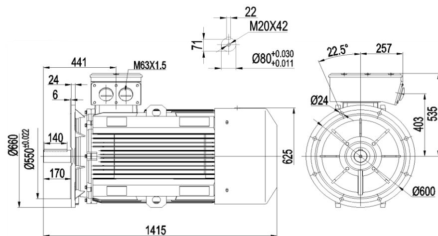
YE4-315L2 200kW(1310kg)
