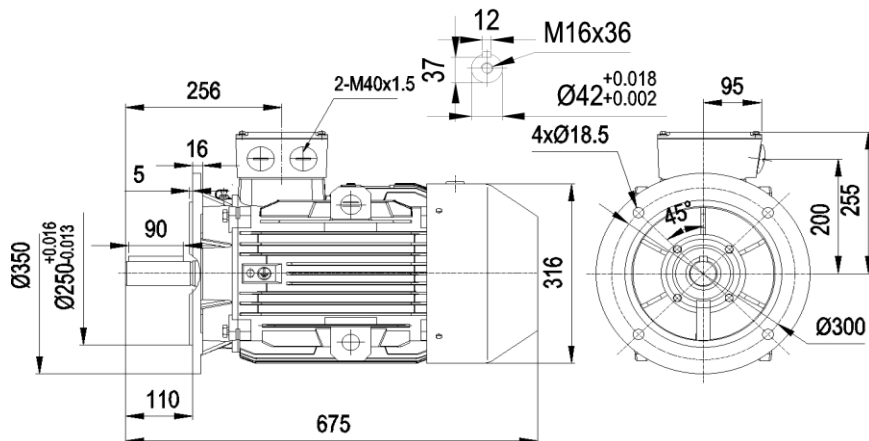
YE4-160M 11kW(145kg)
