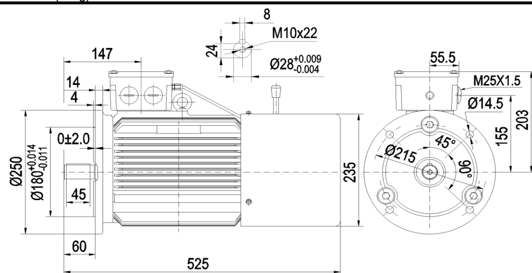
YEB4-112M 3.7kW(74kg)
