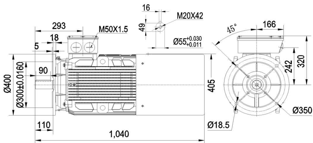
YEB4-200L 30kW(316kg)
