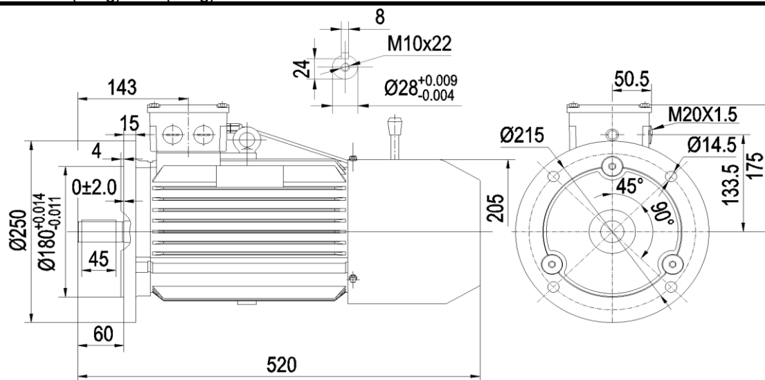
YEB4-100L 2.2kW(61kg)/3kW(65kg)
