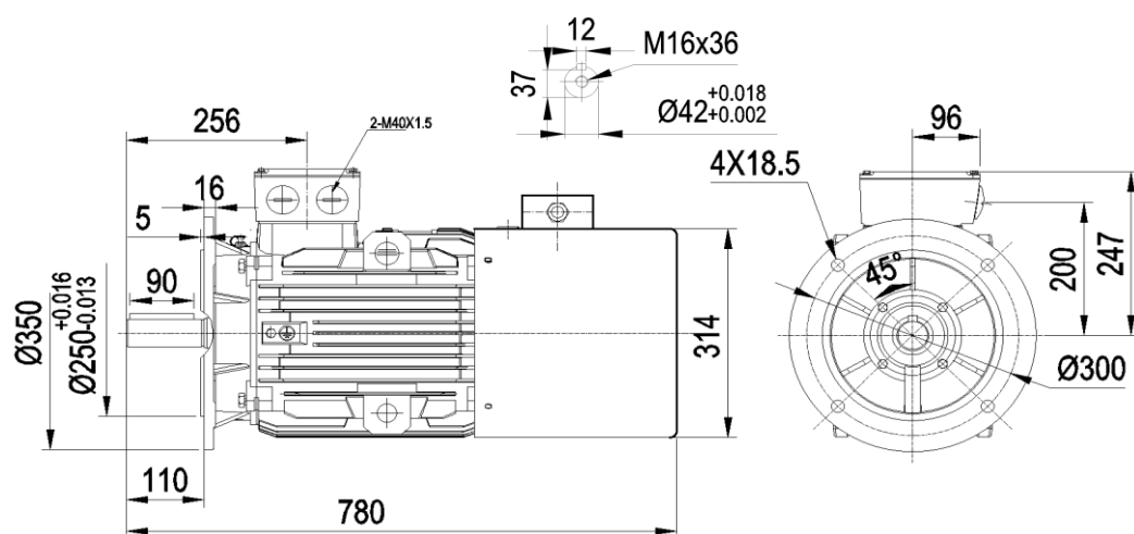
YE4-160M 11kW(145kg)
