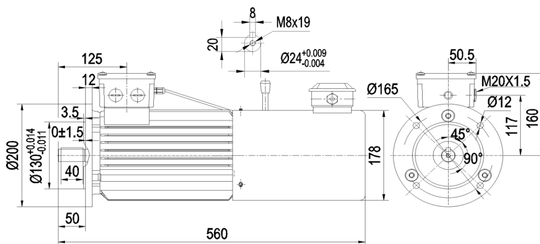
YEB4-90L 1.5kW(49kg)
