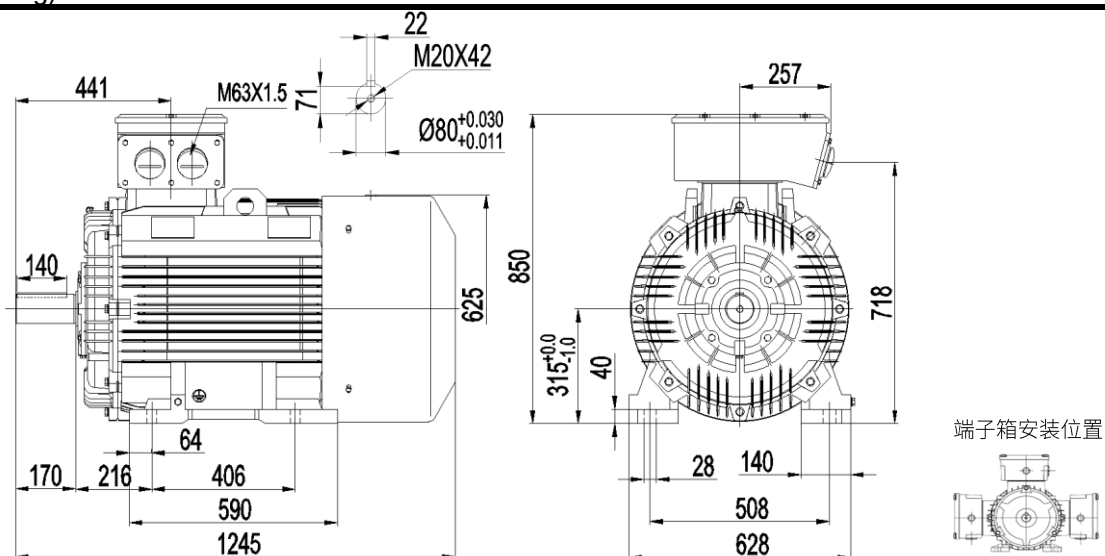
YE4-315M/YE4-315L1 132kW(1070kg)/160kW(1185kg)
