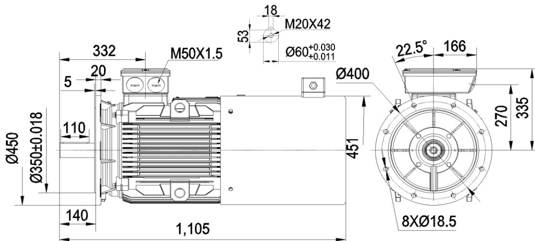
YEB4-225S 37kW(411kg)
