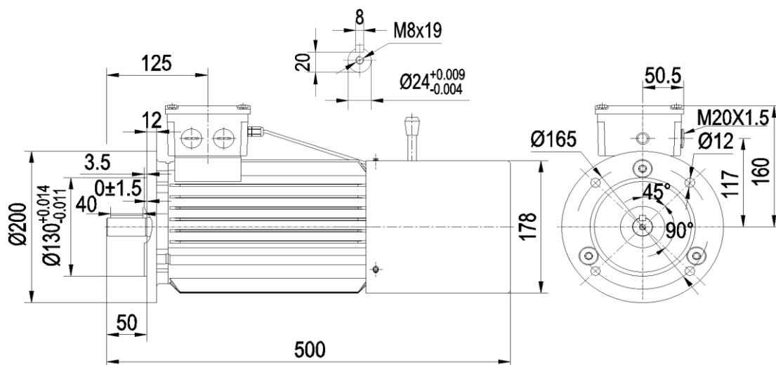
YEB4-90L 1.5kW(49kg)
