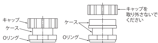
図9 給油栓
