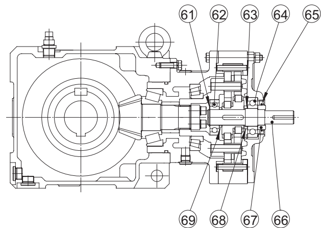
図 10-2 LHY 形(レデューサ) (例: 枠番 4C145-Y1)
