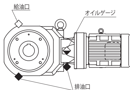
図 8-2 給排油口の位置 (例：ベベル・バディボックス 5 シリーズ LHYM-Y1)
