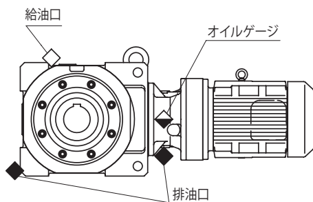
図 8-1 給排油口の位置 (例：ベベル・バディボックス 4 シリーズ LHYM-Y1)
