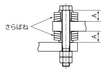
図 5-12 さらばね
