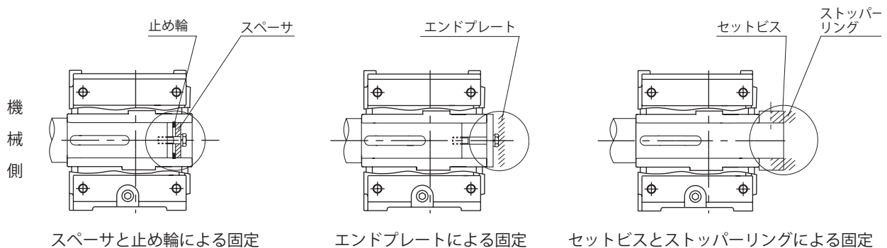
図 5-9 本製品が反機械側に動かない固定方法例
