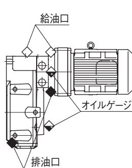
図 8-9 給排油口の位置 (例：ヘリカル・バディボックス EHYM-Y1)
